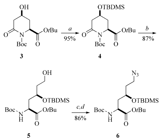
Scheme 1. Reagents and conditions: (a) TBMSCl, imidazole, CH 2 Cl 2 ; (b) NaBH 4 , EtOH; (c) MsCl, DIPEA, CH 2 Cl 2 ; (d) NaN 3 , DMF.
